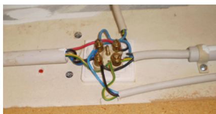
Abzweigdose ohne Berührungsschutz.
