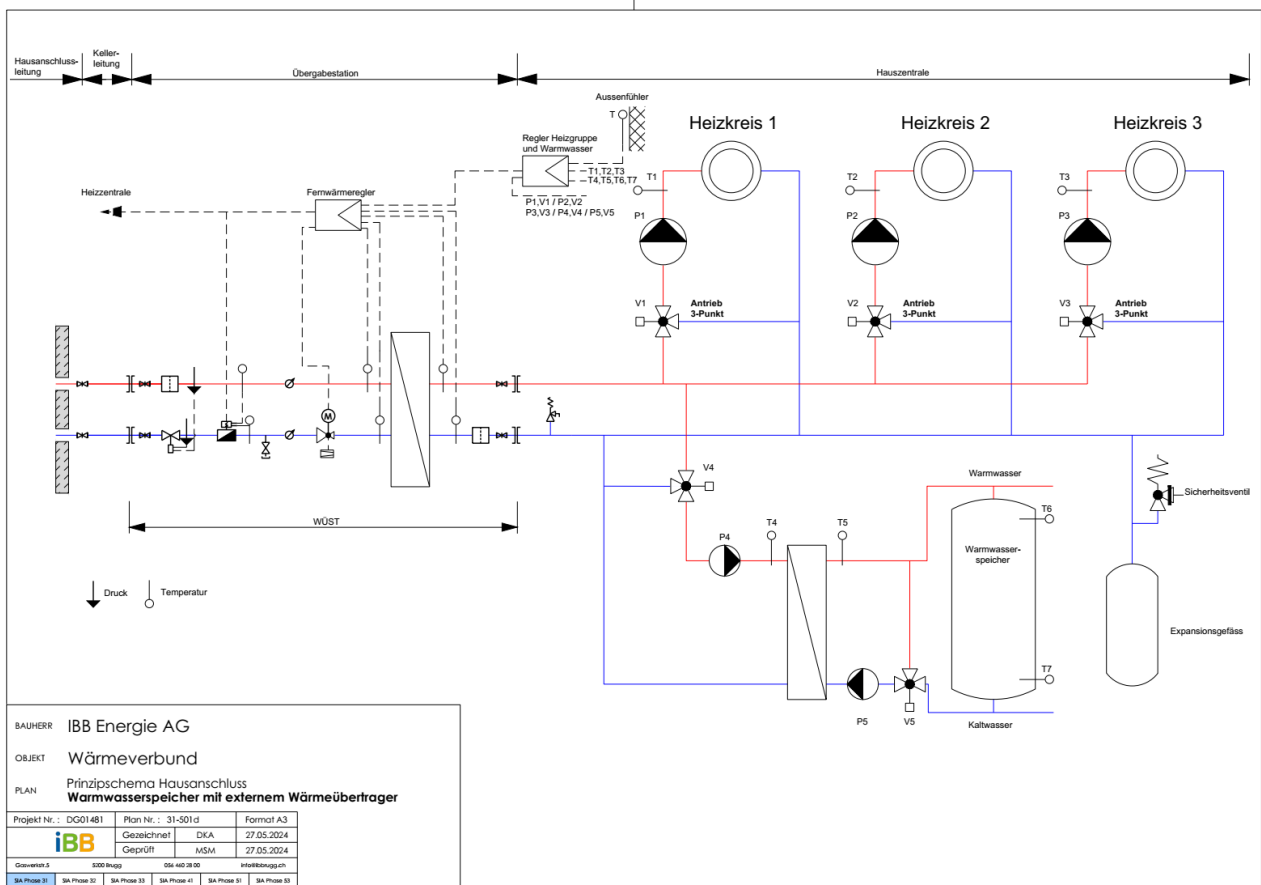
Abbildung 1 Prinzipschema Hausanschlüsse
